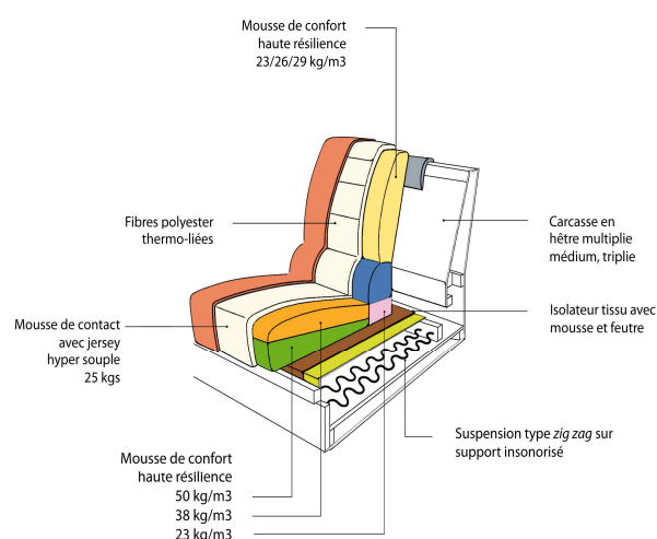
COUPE POUR LE PETIT FAUTEUIL
