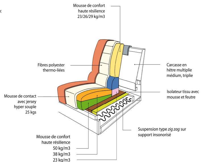
COUPE POUR LE PETIT FAUTEUIL
